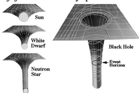
Znázornění zakřivení časoprostoru různě hmotnými objekty
