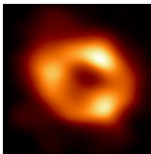
Jediná kdy lidmi pořízená fotografie okolí černé díry v centru Mléčné dráhy (2019)
